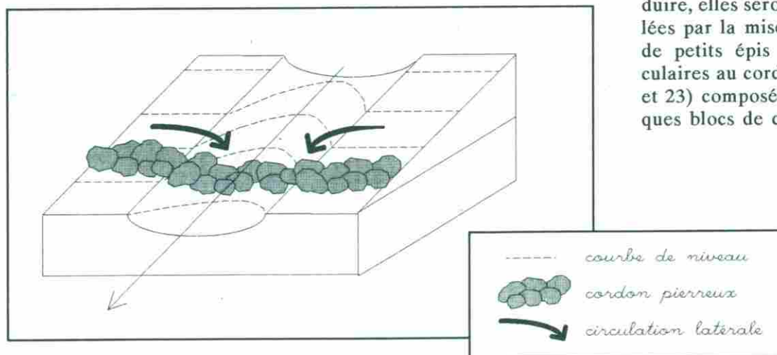
fig.22 : redressement des courbes de niveau lors de la pose du cordon
