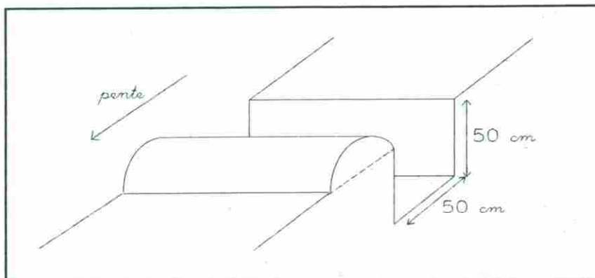
fig. 32 : trouaison; réalisation de la tranchée
