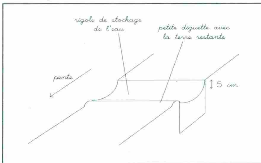
fig. 33 : rebouchage de la tranchée
