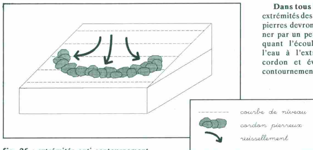
fig. 25 : extrémités anti-contournement
