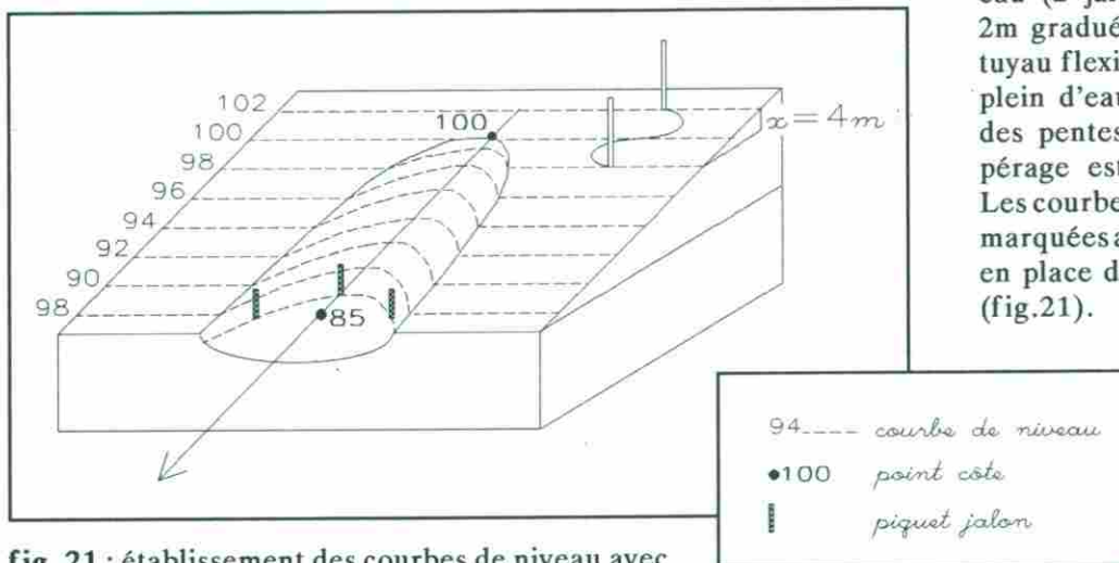
fig. 21 : établissement des courbes de niveau avec un niveau à eau
